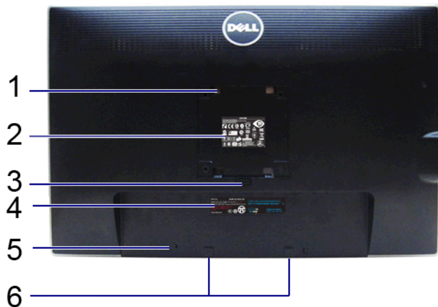
背視圖
